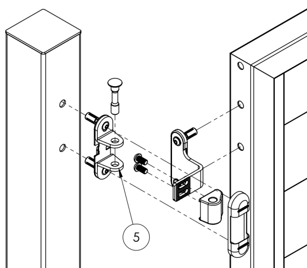
Installation des gonds
